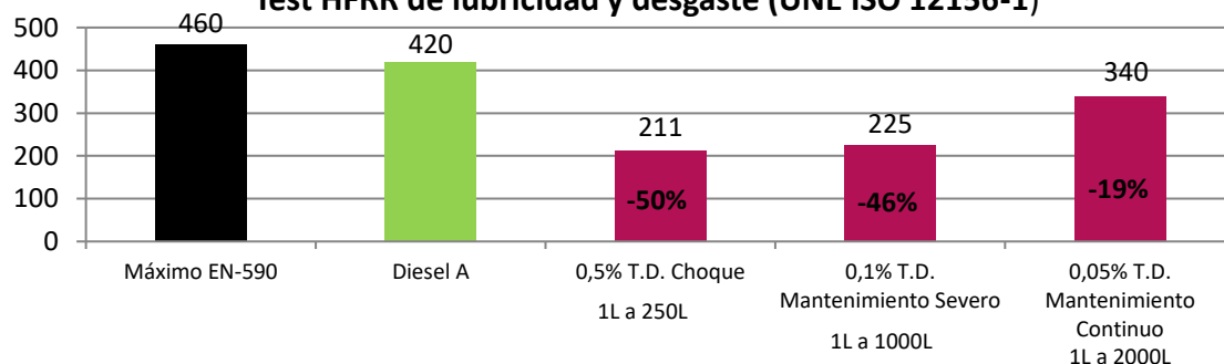
Test HFRR de lubricidad y desgaste (UNE ISO 12156-1)
